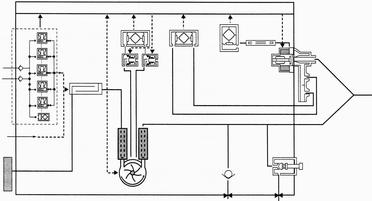
ガスの配流システム
