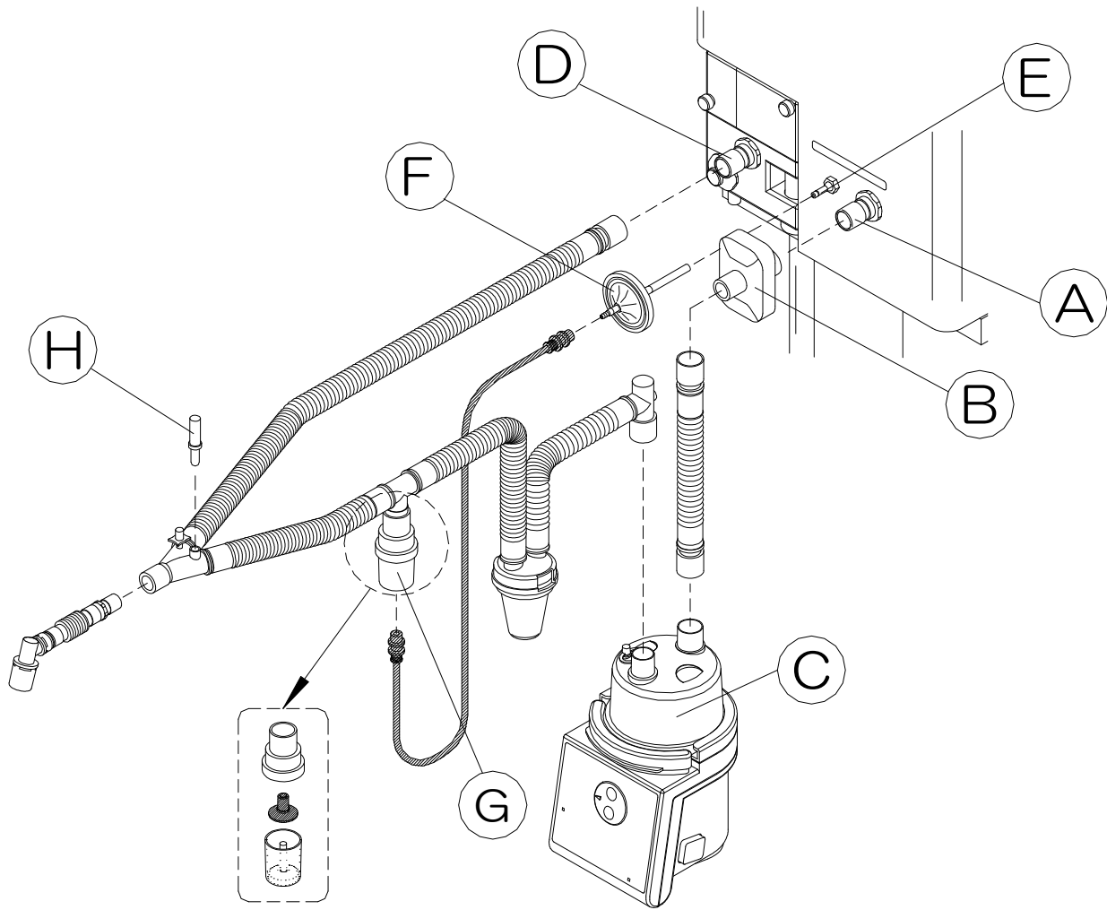
患者回路接続図
