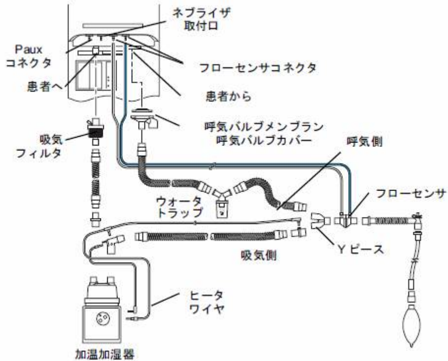
吸気ヒータワイヤを併用する呼吸回路の接続 (小児 / 成人)
