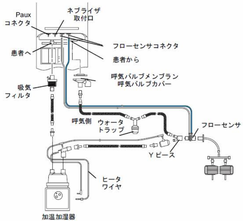
吸気ヒータワイヤを併用する呼吸回路の接続 (新生児)
